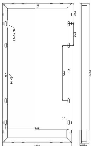
Module Diagram
